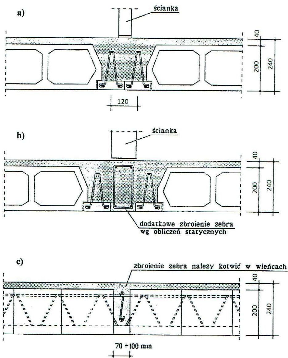
Z3-3. Przykład rozwiązania żeber stropowych a) i b) zebra pod ściankami działowymi, równoległymi do belek, c) zebro rozdzielcze.
